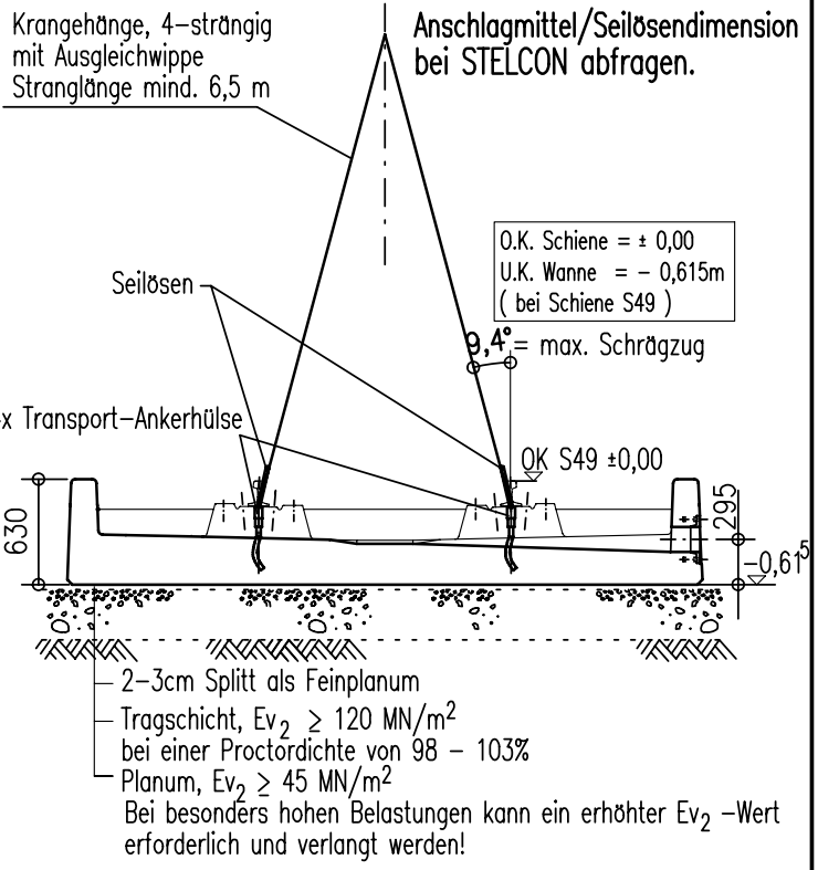
QUERSCHNITT dargestellt: EW 5000/3800 S49/S54
