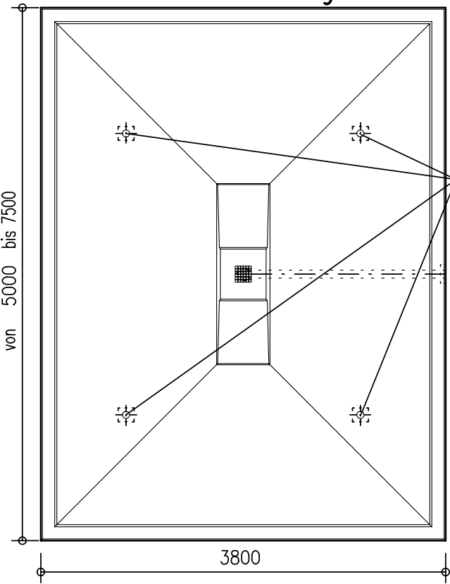
DRAUFSICHT dargestellt: Tragwanne 5000 x 3800
