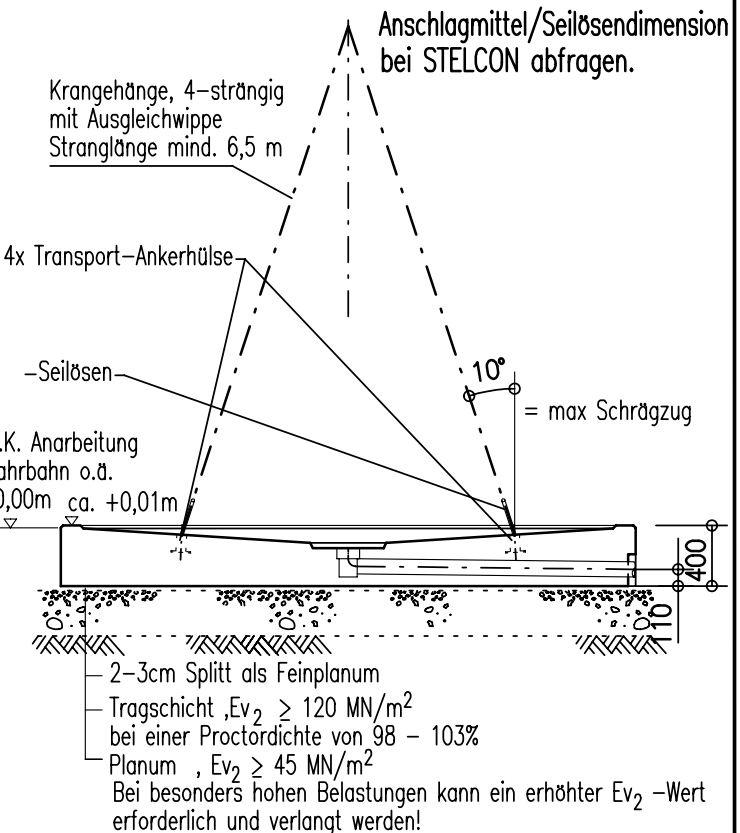
QUERSCHNITT dargestellt: Auffangwanne 5000 und 7500 (vormals Zeichnung Nr.P98/228/1a)
